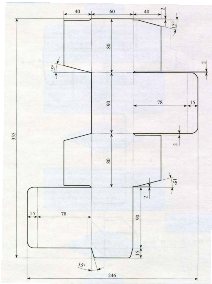
Сл. 7. Детаљ цртежа расклопљене кутије
