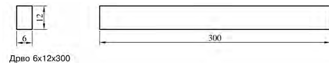
Сл. 11. Дрво 6 x12 x 300
