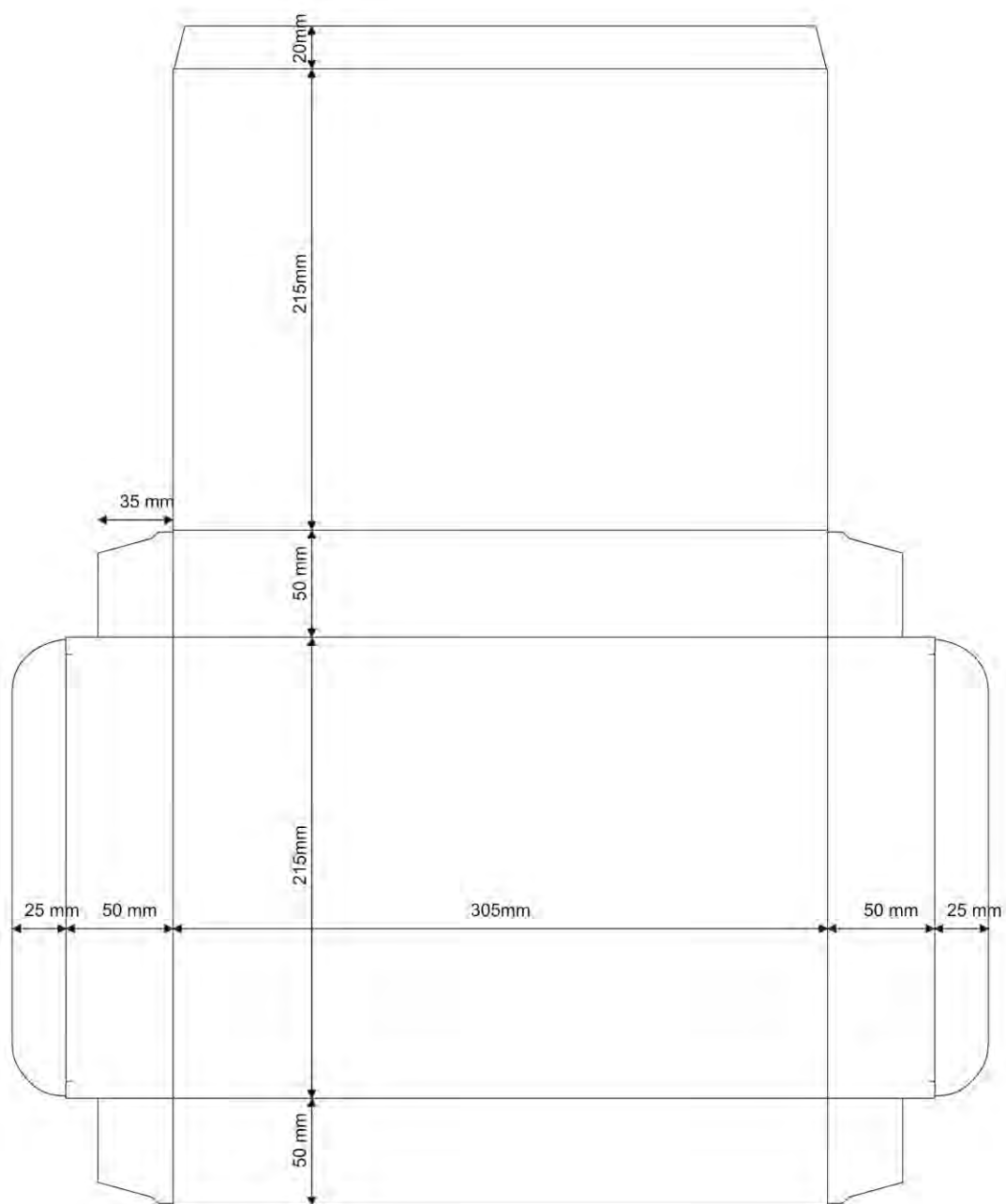
Цртеж, шема израде кутије за збирку материјала за техничко и информатичко образовање за 5. разред основне школе
