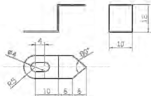
Сл. 13. Детаљ контакта
