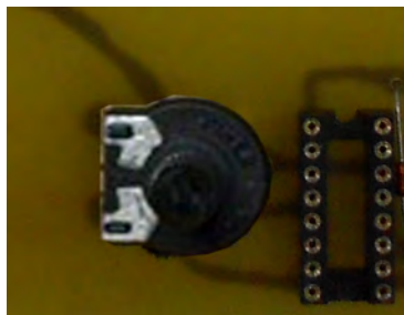
Сл. 6. Потенциометар – тример
