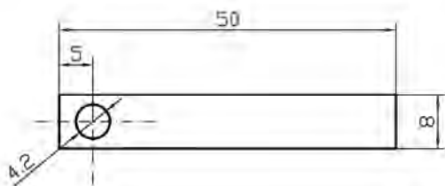
Сл. 16. Котва ( бат ) зујалице
