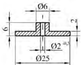
Сл. 17. Деталъ диска електромотора
