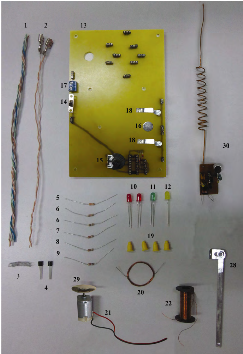
Сл. 1. Материјал за извођење вежби за техничко и информатичко образовање
