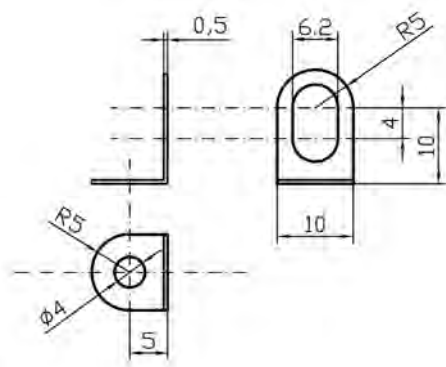
Сл.12. Држач електромагнета
