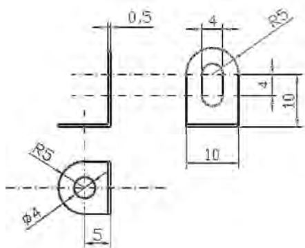
Сл. 15. Држач зујалице
